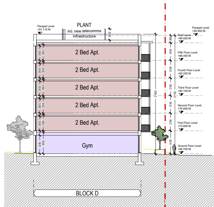
Block D - Section DD
